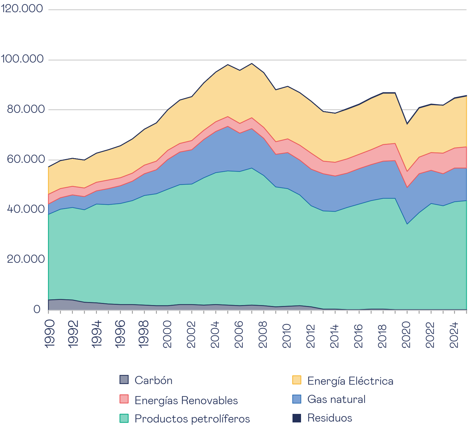
Figura 1. Consumo de energía final en España por fuentes energéticas
