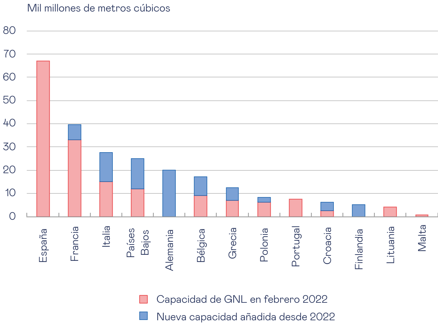
Figura 2. Capacidad de regasificación de GNL en la Unión Europea, por países
