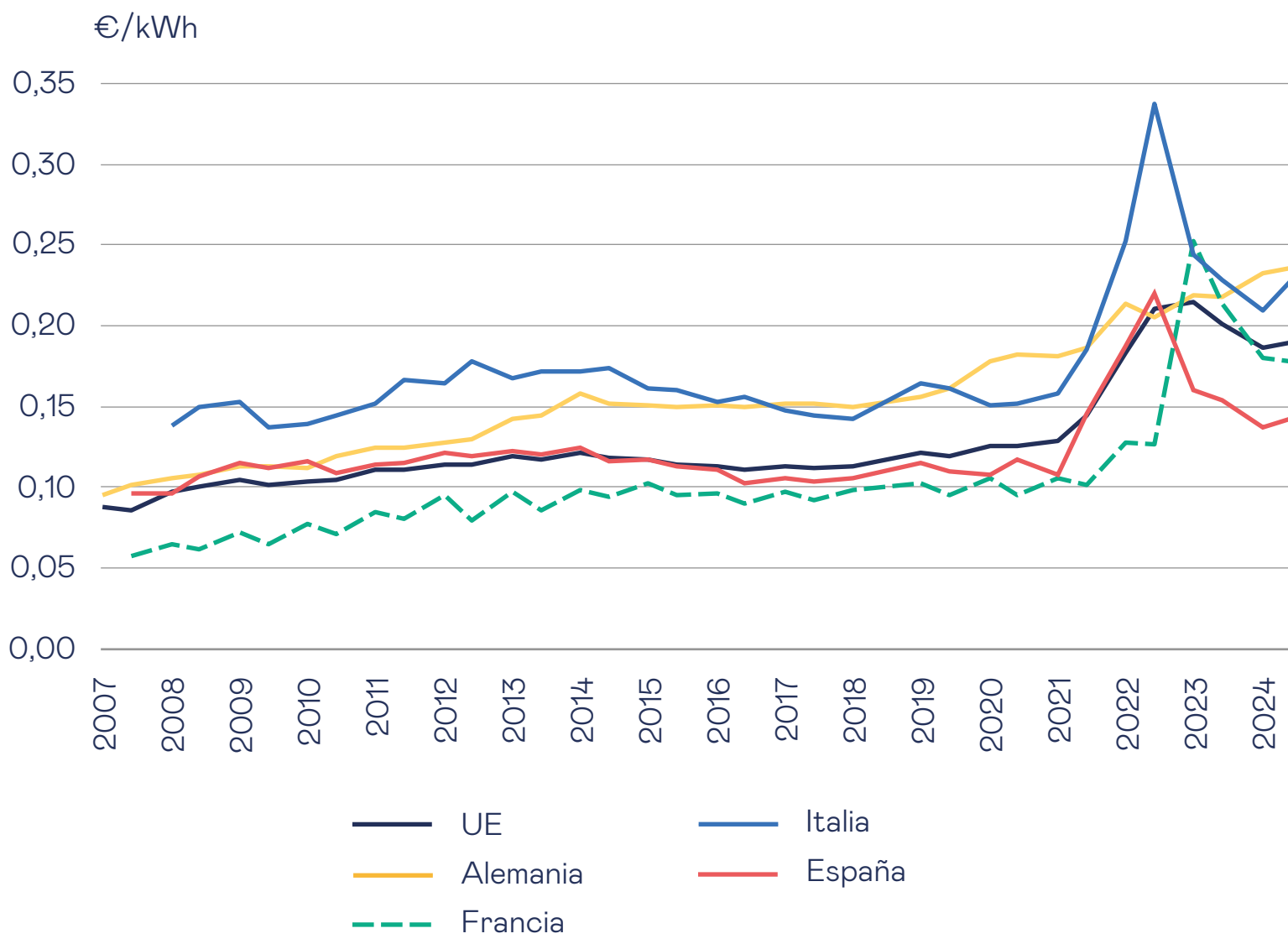
Figura 4. Evolución del precio minorista de electricidad para usos industriales en la UE y las principales economías europeas
