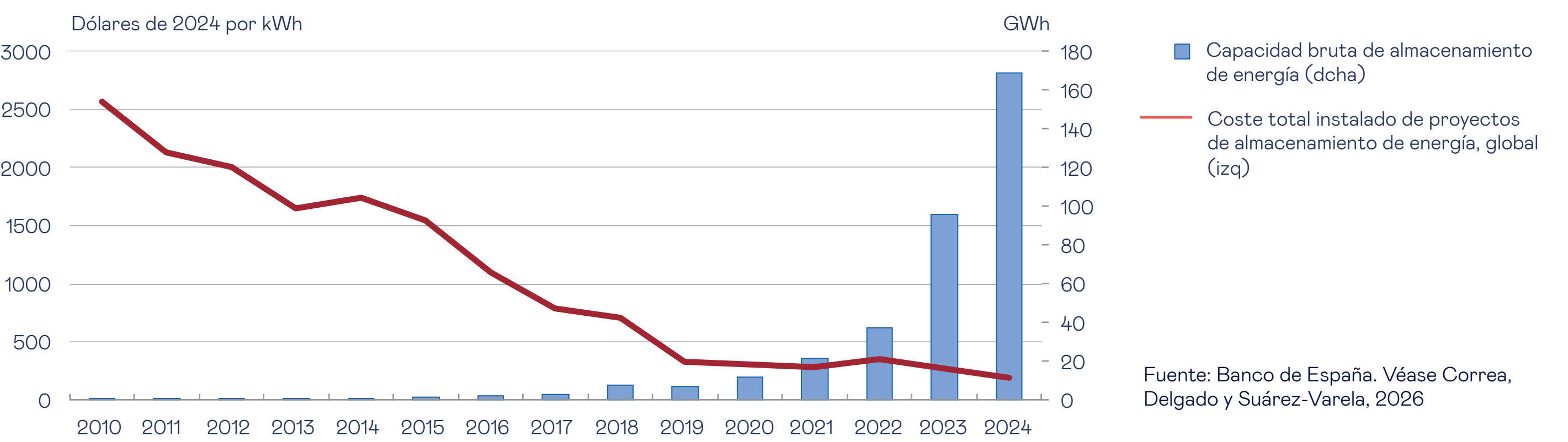
Figura 8. Capacidad bruta de almacenamiento instalada y costes totales de instalación de proyectos de almacenamiento de electricidad, 2010–2024
